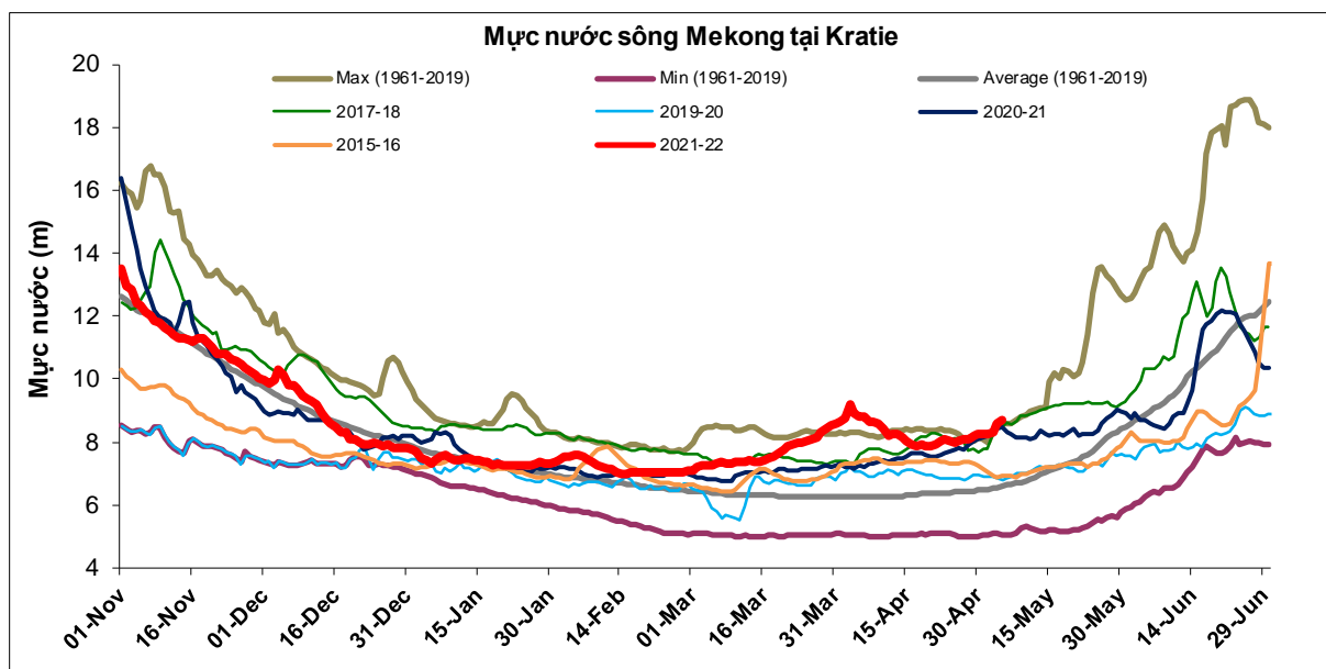
Hình 3. Diễn biến mực nước về qua trạm Kratie, cập nhật ngày 05/5/2022
