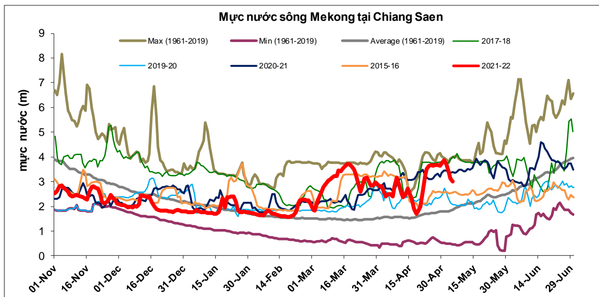
Hình 2. Diễn biến mực nước tại Chiang Saen –Thái Lan, cập nhật 05/5/2022
