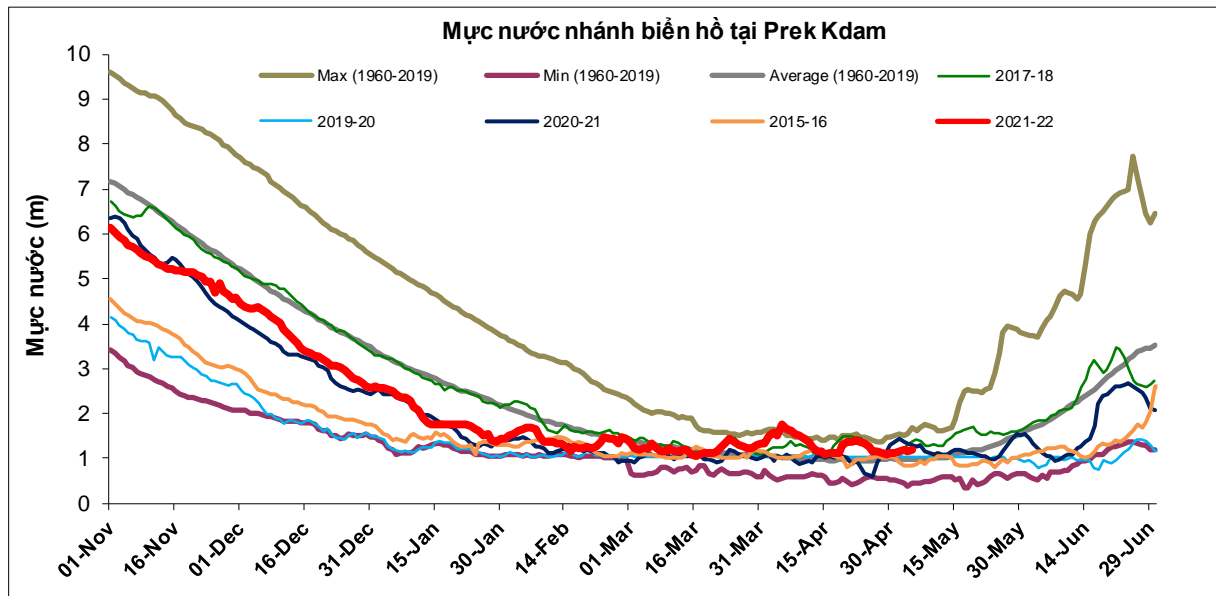
Hình 1. Diễn biến mực nước trạm Prek Kdam - Biển hồ, cập nhật ngày 05/5/2022
